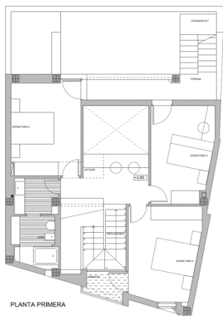
PLANTA PRIMERA
