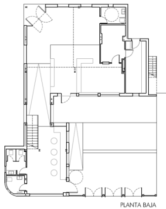
PLANTA BAJA
