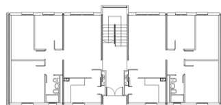
PLANTA TIPO 3D ESTADO REFORMADO. E:1/200
