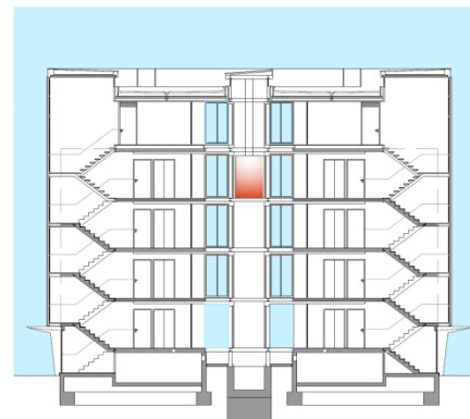
SECCION TRANSVERSAL ESTADO REFORMADO E:1/200
