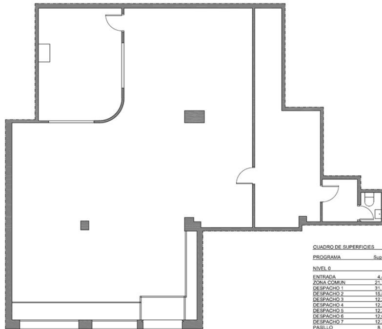
PLANTA BAJA, ESTADO PREVIO.
