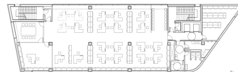
Planta tercera
