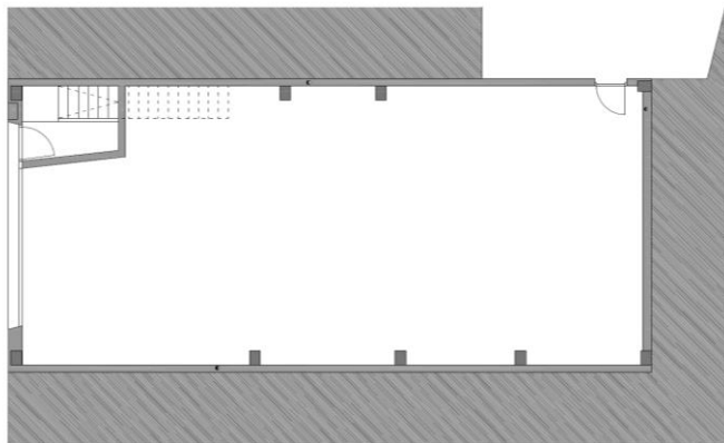
PLANTA BAJA
