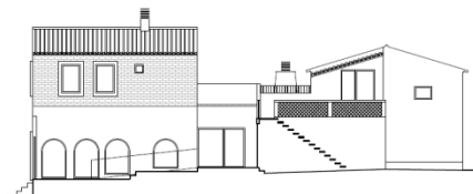
SECCIÓN LONGITUDINAL L5. ALZADO ESTE
