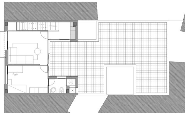
PLANTA SEGUNDA
