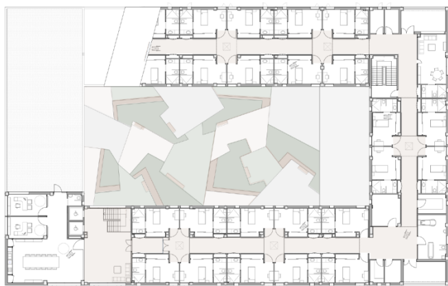
PLANTA PRIMERA
