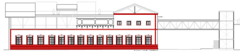
ALZADO CALLE VITERBO
