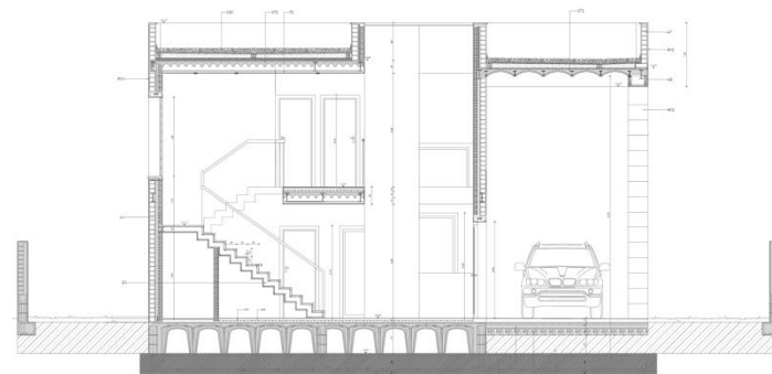
SECCIÓN TRANSVERSAL
