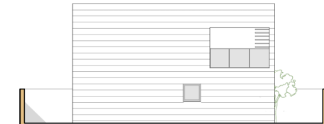
ALZADO OESTE
